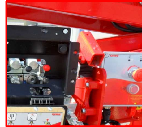
Afbeelding 18: bedieningspost handpomp.
